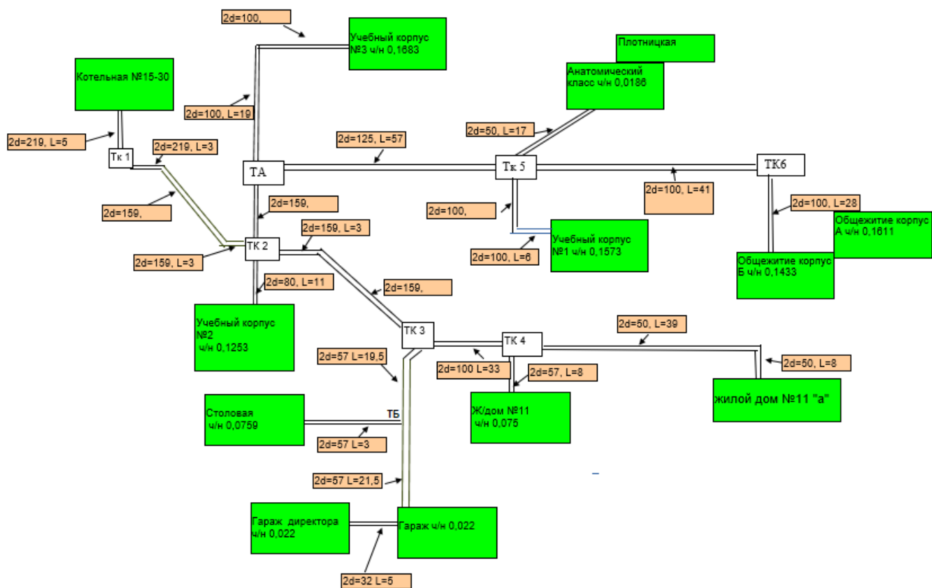
1.3.2.18 Схема тепловой сети Котельной №15-30
